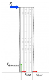
Charge sur les ancrages et Steel Strong-Wall
