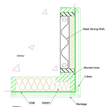
Exemple d'intégration de Strong-Wall dans un angle
