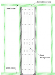
Exemple d'intégration de SSW avec lisses haute et basse
