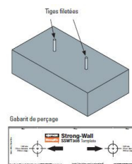
Etape 1 - Mise en place des tiges filetées.
