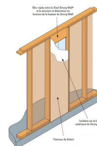
Etape 4 - Mise en place d'un bloc rigide entre le SSW et la structure.
