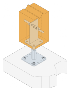
Fixation d'un poteau par broches
