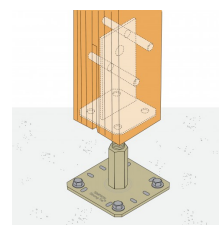
Fixation d'un poteau par broches
