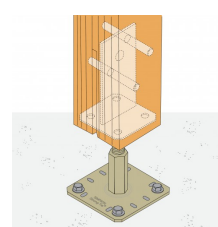
Bevestiging 2 pennen
