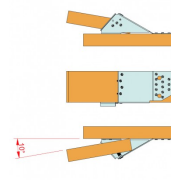
S1030 à 10° avec vis CSA ou pointes CNA
