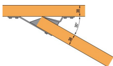
S1530 - Connexion de fermettes avec un angle de 30°
