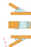
S1030 à 30° avec pointes CNA
