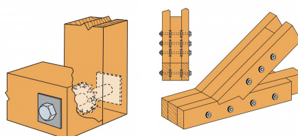
Inspending van een spant
