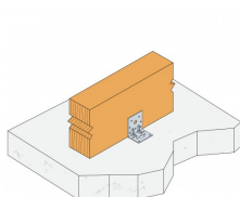
Bevestiging hout op harde ondergrond Balk
