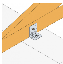
Bevestiging hout op hout Balk op balk
