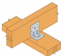
Bevestiging hout op hout Balk op balk
