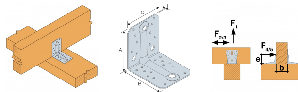
Fixation bois/bois
