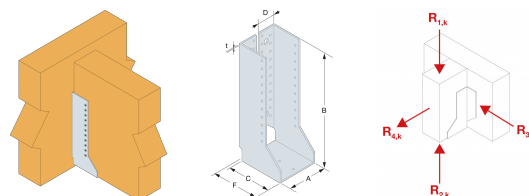
Valeurs Caractéristiques - Bois sur bois - Clouage total
