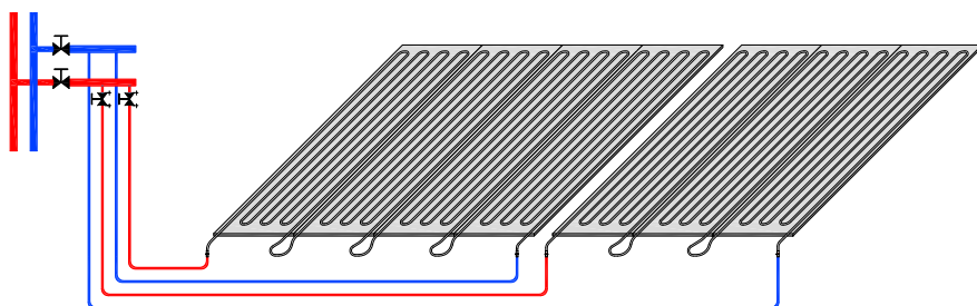
Combinatie van platen aangesloten op verdeler
