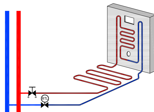
Aansluiting toiletmodule op CV-systeem
