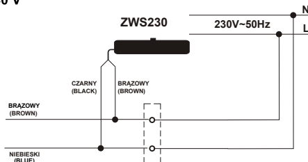
Schemat elektryczny Wiring diagram
