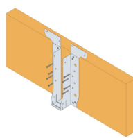
Fixation par les brides latérales sur un support bois massif
