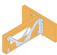
Fixation d'une poutre métallique ajourée par les brides latérales sur un support bois massif
