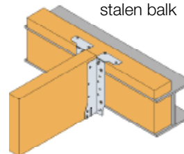
Massieve balk op stalen balk
