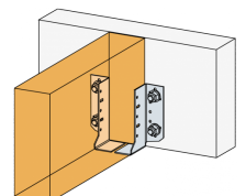
Mise en œuvre SJHR + SJHL sur béton
