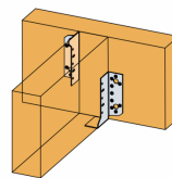
Mise en œuvre SJHR + SJHR-F sur bois
