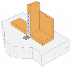
Uitvoeringswijze 1 1 onderregel 45 mm
