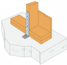
Uitvoeringswijze 2 2 onderregels 45 mm
