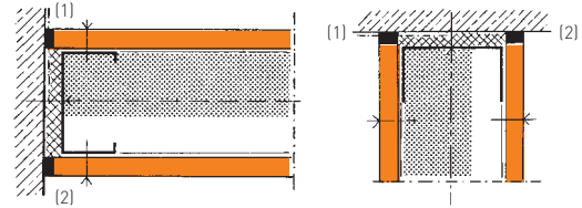
Raccords au mur et au plafond d'une double couche de plaque FERMACELL.
