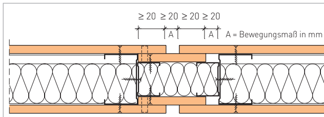
FERMACELL Montagewand, einlagig beplankt, F 30-A/F 60-A. Bewegungsfuge mit Plattenstreifen
