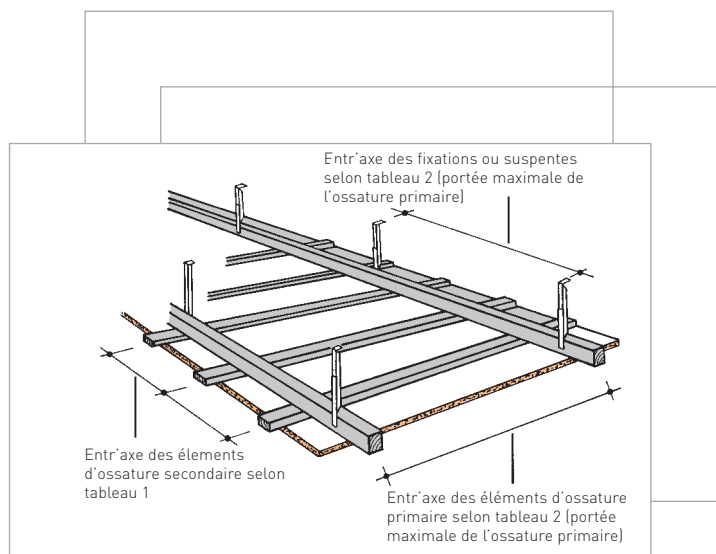
Figure 16 : Exemple de montage de suspentes, ossature primaire/lattage et secondaire/contre-lattage.
