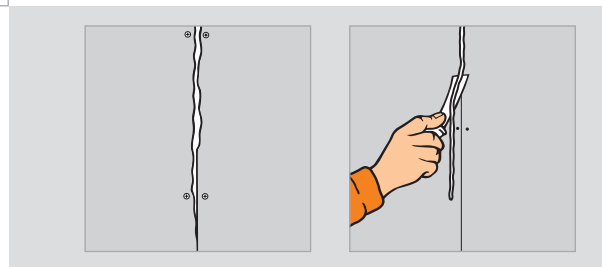
Figure 15 : Etape 5 Après séchage et expansion de la colle (12 à 36 heures) ractler les bavures de colle et araser les passages de tête de vis à l'aide d'un couteau à mastic ou d'une spatule à bords arrondis.
