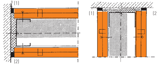
Raccords au mur et au plafond d'une double couche de plaque FERMACELL.
