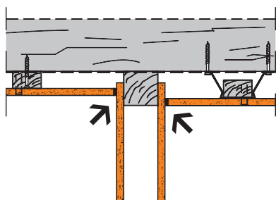
Raccord à l'angle comme plafond horizontal ou rampant cf. page 19
