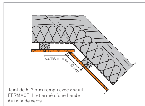
Figure 17 : 1. Joint classique avec bande
