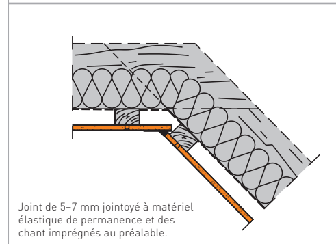
Figure 19 : 3. Joint à élasticité permanente (par exemple en acrylique)
