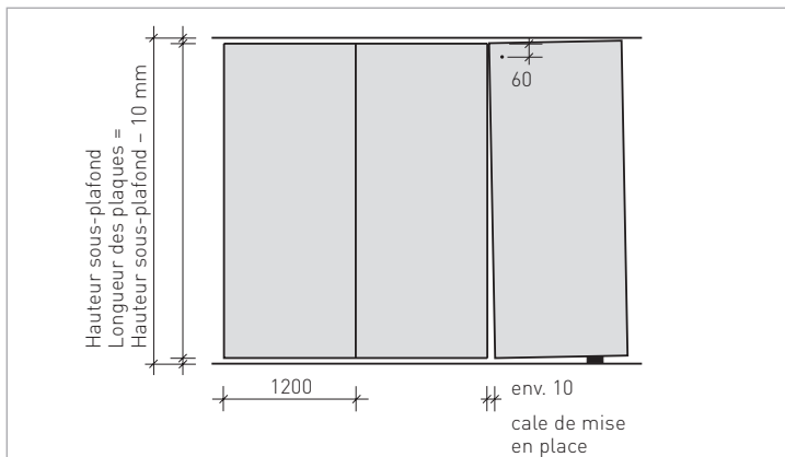
Figure 13 : Etape 3 Positionner la plaque suivante sur une cale de façon à ce que son angle supérieur touche la première plaque tout en laissant une fente verticale d'un chant à l'autre (ceci suppose que la longueur des plaques soient inférieure d'environ 10 mm à la hauteur sous-plafond). Solidariser l'angle supérieur de la seconde plaque avec une première vis. Retirer ensuite la cale. La plaque FERMACELL va pivoter de par son propre poids autour de l'angle supérieur et écraser le cordon de colle. Le joint ainsi réalisé ne doit pas dépasser 1 mm de large.
