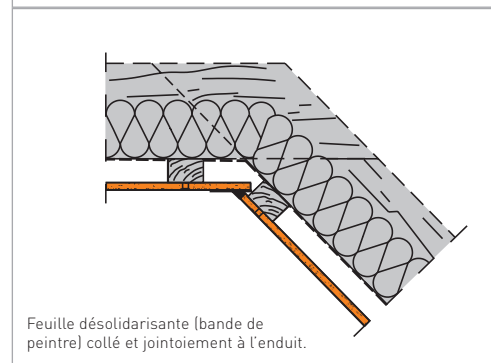
Figure 18 : 2. Jointolement avec feuille désolidarisante
