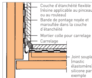
Figure 26 : Raccord vertical format un angle rentrant en zone soumise aux ruissellements et projections.
