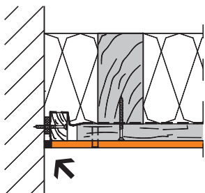
Raccord à l'angle avec joint à élasticité permanente
