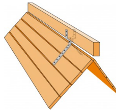
Bevestiging volgens helling van het dak (in situ plooibaar
